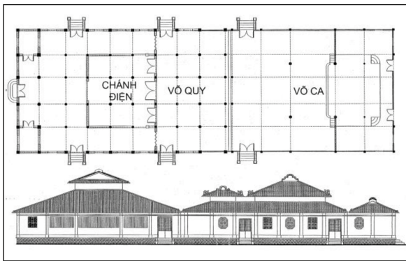
Hình 11. Bản vẽ kiến trúc Đình Tân Giai [10]
