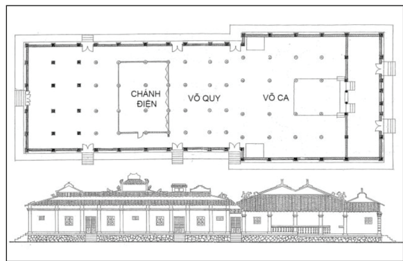
Hình 10. Bản vẽ kiến trúc Đình Tân Hoa [10]
