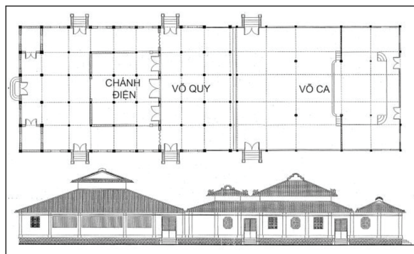
Hình 12. Bản vẽ kiến trúc Đình Tân Ngãi [10]
